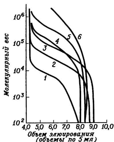
Р и с. 5.4. Зависимость между молекулярным весом и объемом элюирования для различных типов пористого стекла (растворенные вещества: полистиролы; подвижная фаза: толуол [17]).
