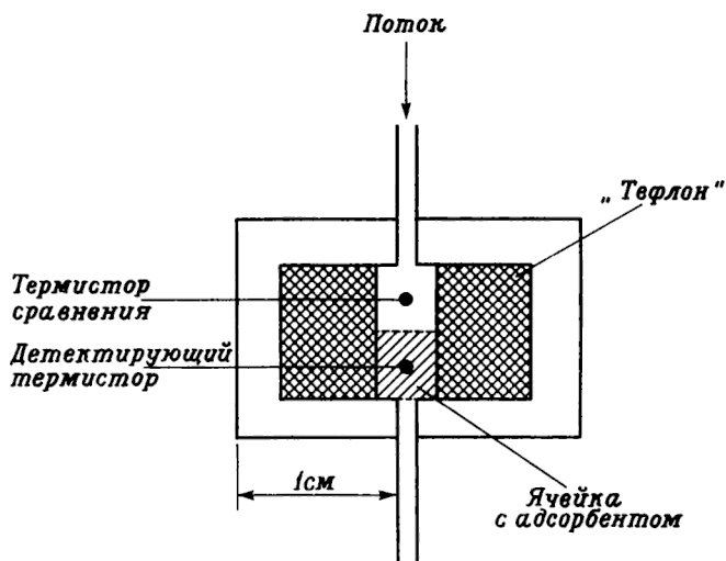
Р и с. 7.12. Детектор по теплоте адсорбции.
