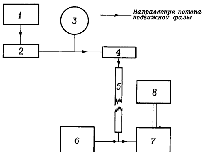
Р и с. 1.2. Схема колоночного хроматографа. 1 - резервуар с элюентом; 2 - насос или другой источник давления; 3 - манометр; 4 - устройство для ввода пробы; 5 - колонка; 6 - коллектор фракций; 7 - детектор; 8 - самописец с линейной диаграммой.
