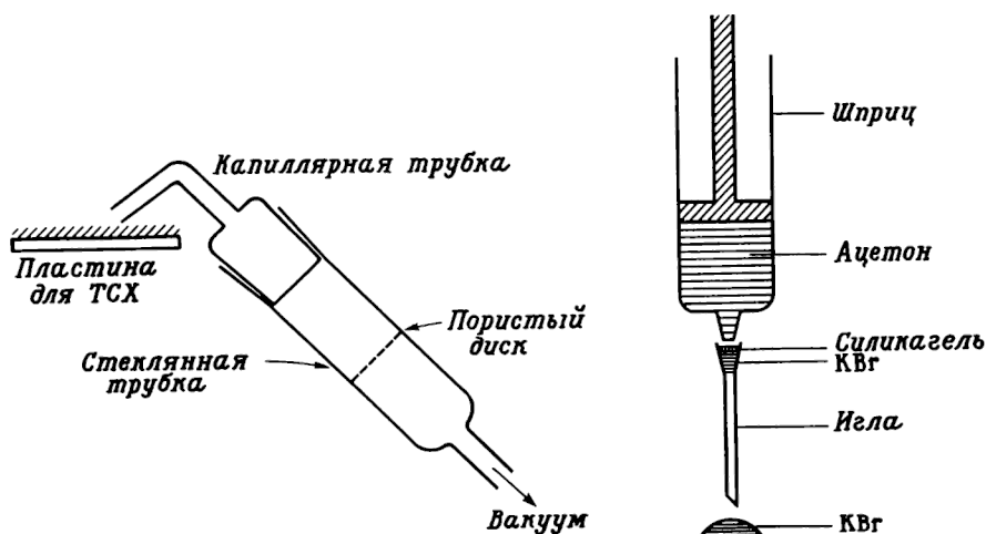
Р и с. 6.13. Устройство для удаления адсорбента с пластинки для ТСХ.
