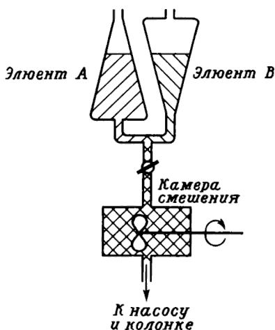
Рис. 7.8. Стеклянное устройство для создания линейных градиентов элюента.
