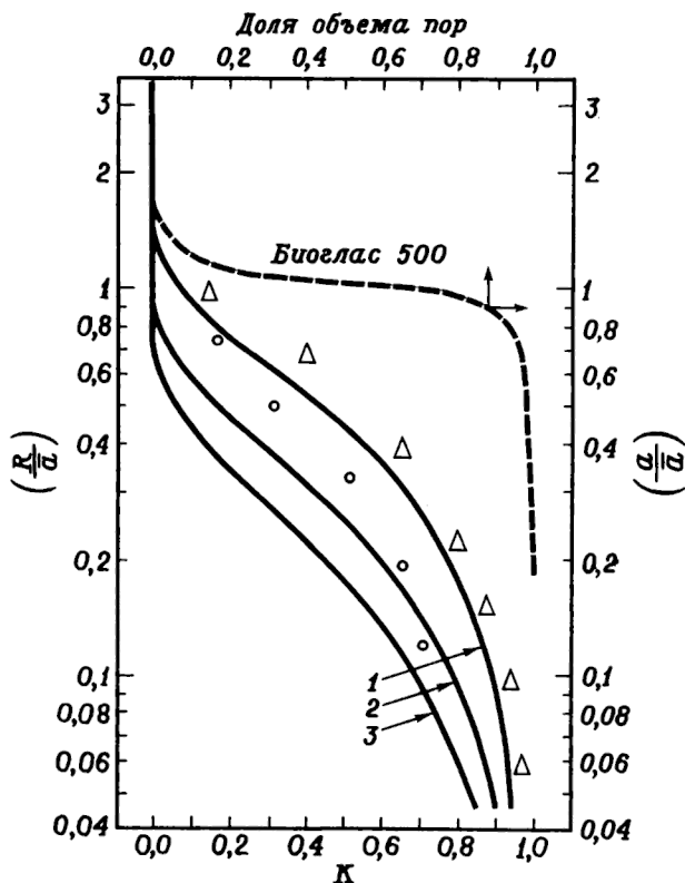
Р и с. 5.3. Данные, полученные при разделении на неподвижных фазах с различным распределением пор по размерам, и теоретически кривые Казассы [3]. Неподвижная фаза: \Delta биоглас 500, O биоглас 200; форма пор: 1 – щелевидные, 2 – цилиндрические, 3 – сферические.
