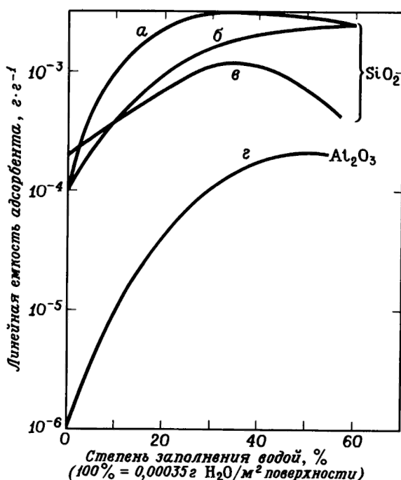
Р и с. 3.4. Зависимость линейной емкости адсорбента от типа адсорбента и относительной дезактивации водой [2].
