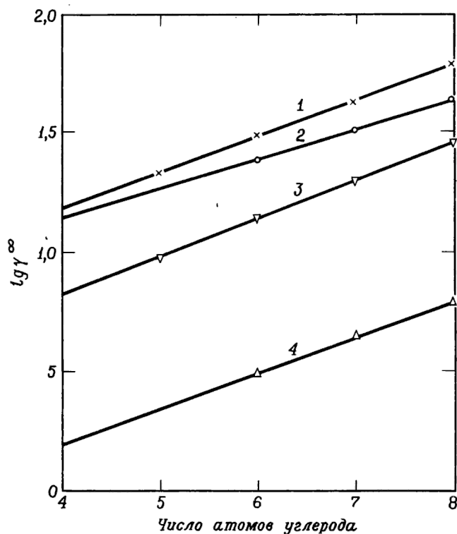
Р и с. 4.1. Коэффициенты активности в ацетонитриле, определены методом распределительной хроматографии при 25°C. 1 – n-алканы; 2 – монозамещенные циклогексаны; 3 – олефины-1; 4 – монозамещенные алкилбензолы.
