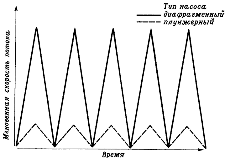
Рис. 7.3. Профили недемпфированного потока, создаваемого насосом.
