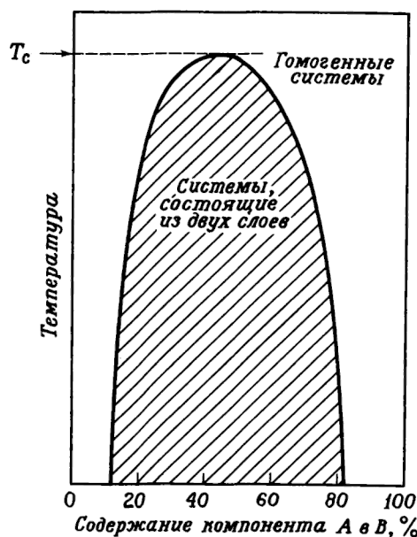
Рис. 4.3. Критическая температура растворения бинарной смеси.
